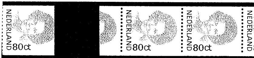
Afbeelding 1: Las met rood plakband bij Beatrix, 80 cent.
