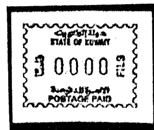
Afb.18 0000-waarde
