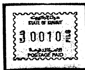
Afb.17 AS-Koeweit
