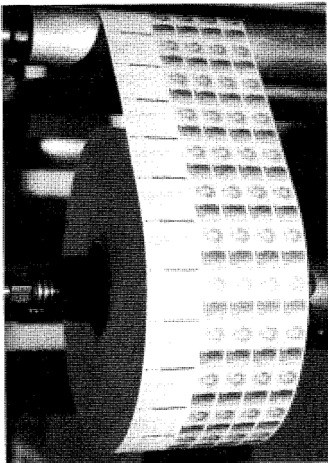
3 - Rol met de zegelinhouden voor boekje 27 b op de boekjesmachine.
