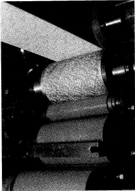
1 - Drukcilinder voor het kaftmotief en een gedeelte van de kaftbaan.
