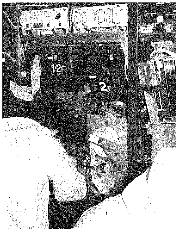
Afb. 16 Binnenwerk CROUZET-automaat let op blanco rol; geldwisselaars; schakelaar linksboven in TEST-stand
